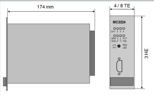
Abmessungen
